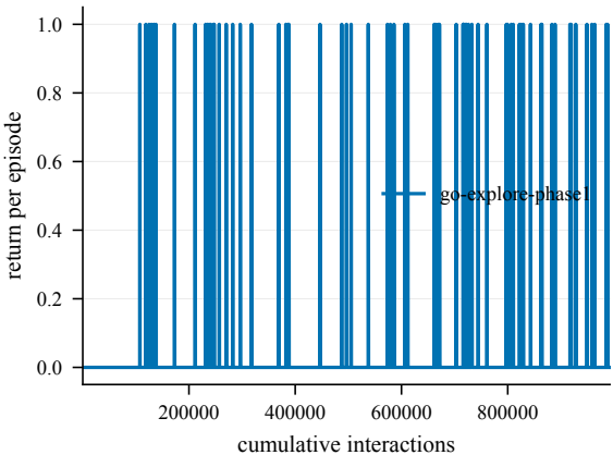
Return -- TopKlein-50@4000
