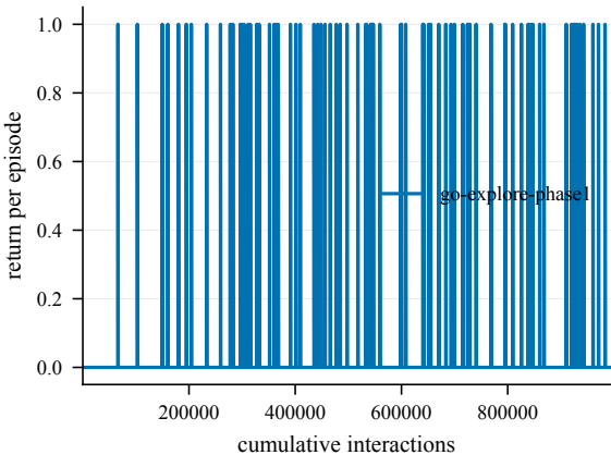
Return -- TopKlein-50@4001
