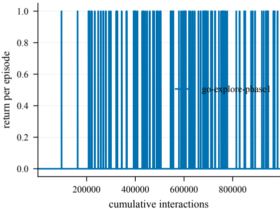
Return -- TopMobius-50@4001
