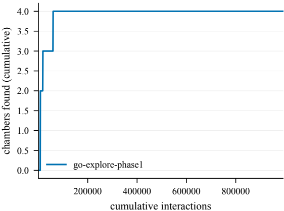
Chambers -- TopMobius-50@4002
