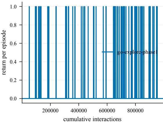
Return -- TopRP2-50@4000
