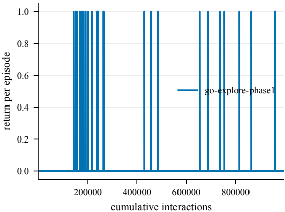
Return -- EpicChase6-110@12
