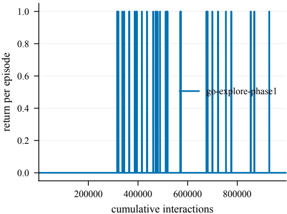
Return -- EpicChase6-110@16
