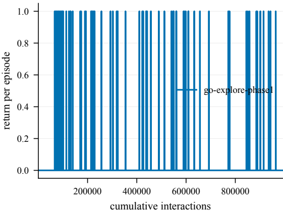
Return -- EpicChase1-60@2
