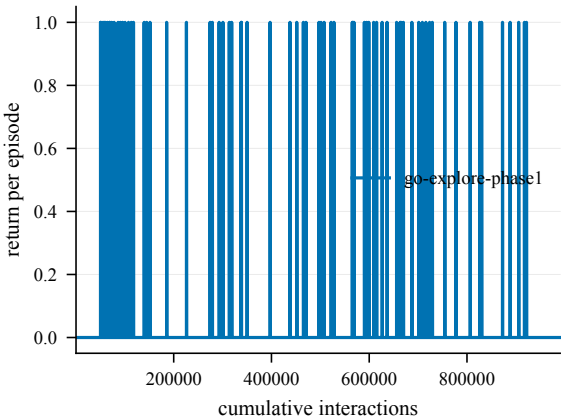
Return -- EpicChase1-60@6
