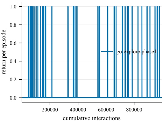
Return -- EpicChase3-70@3
