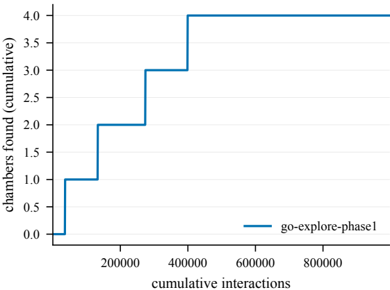
Chambers -- EpicChase4-90@2
