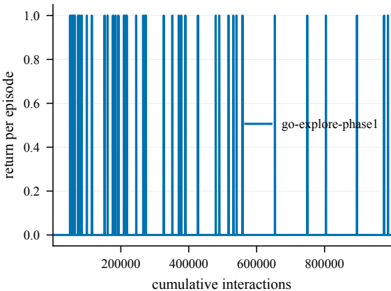
Return -- EpicChase6-110@2
