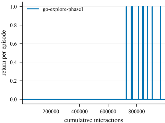
Return -- EpicChase8-120@4
