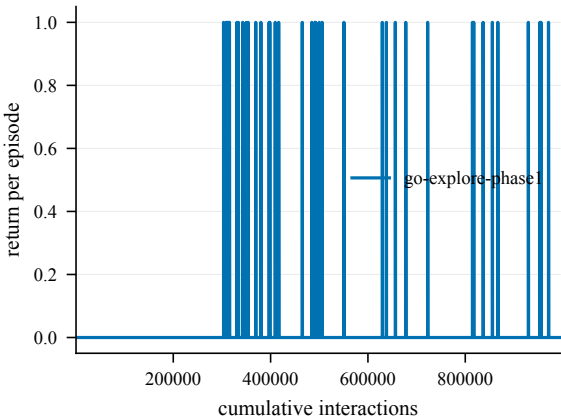
Return -- EpicChase8-120@7
