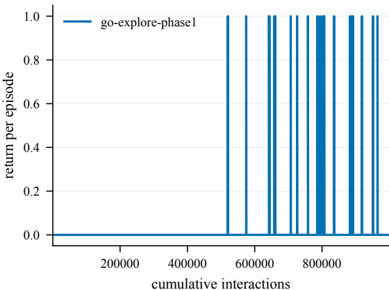
Return -- EnlargedChamberCount5-100@4
