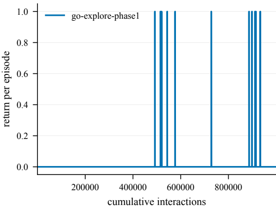
Return -- EnlargedChamberCount8-150@4
