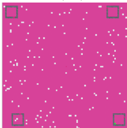
TE (ricci)
