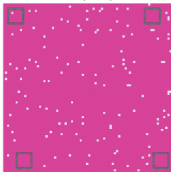
TE (none)
