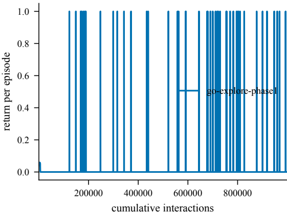
Return -- ClownChase
