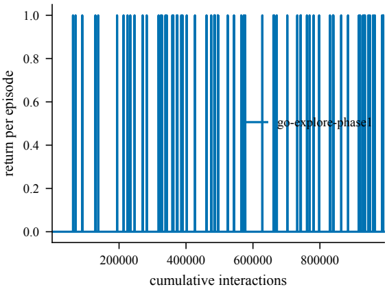
Return -- TopRP2-50
