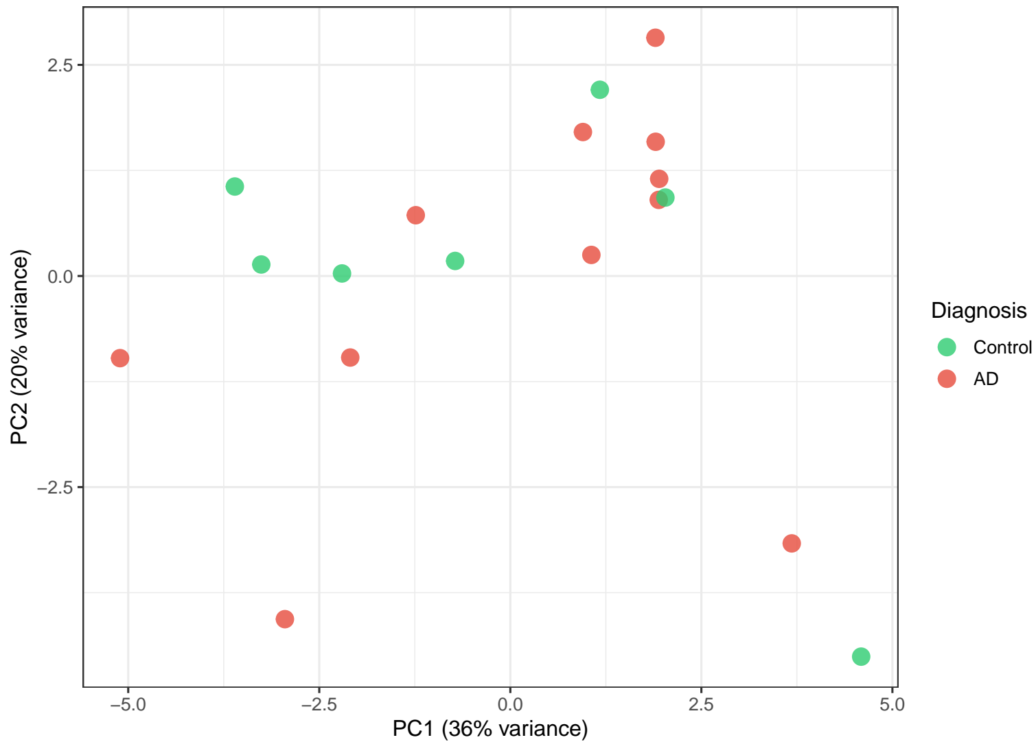
PCA of TE Expression
