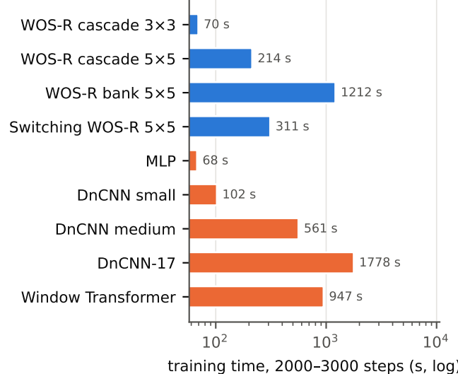
(d) Training time
