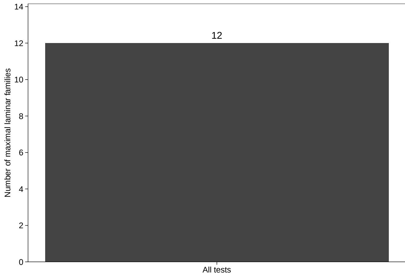
Teotitlán del Valle Zapotec (verbal) (teot1238_verbal): all tests
