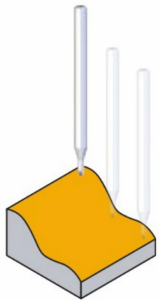
使用球头铣刀进行曲面加工 3D milling by ball end mill
