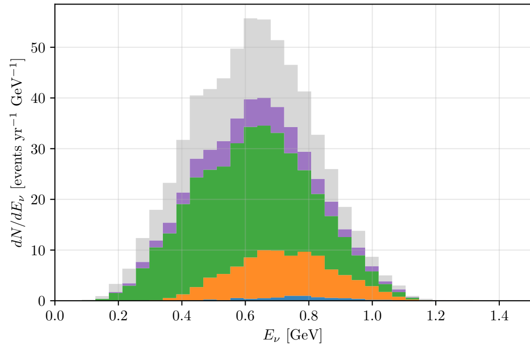
PA: \nu_e on Ar40
