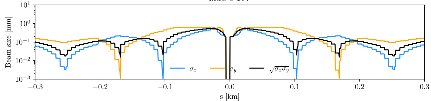
MuC-3-TeV
