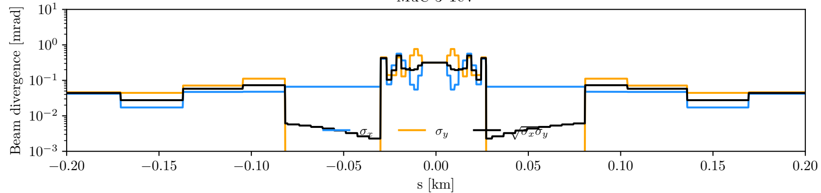
MuC-3-TeV
