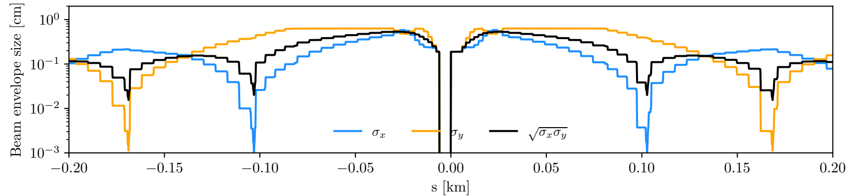
MuC-3-TeV
