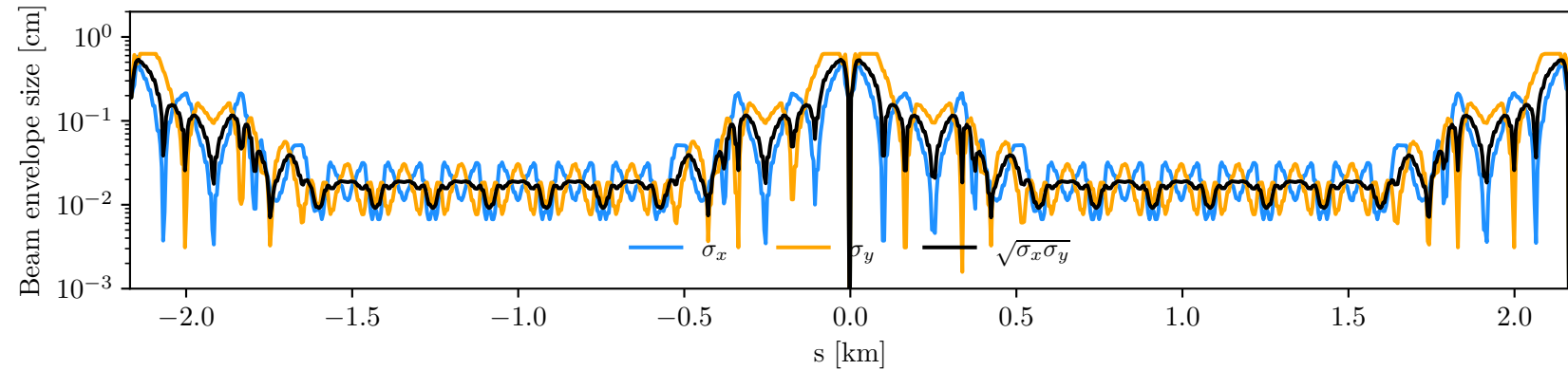
MuC-MuC-3-TeV
