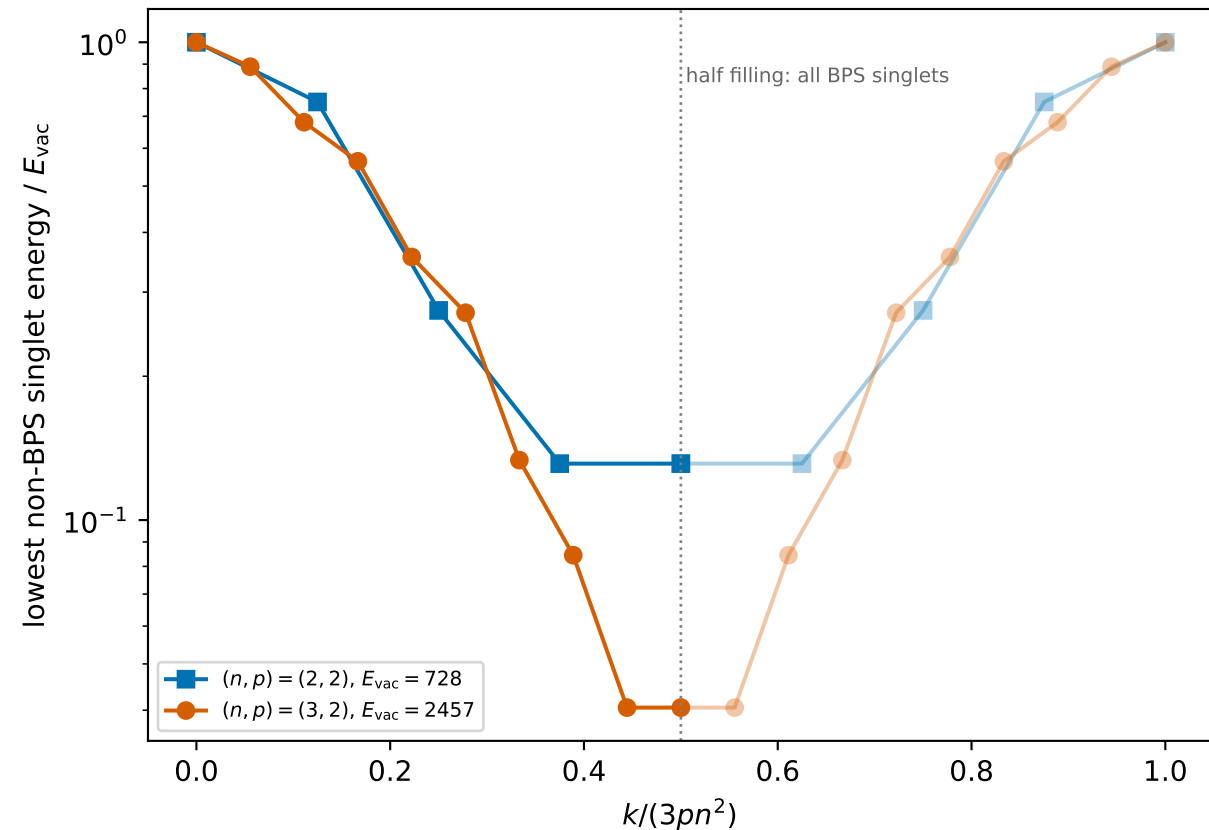
(d) next rank, p = 2 : singlet gap per degree
