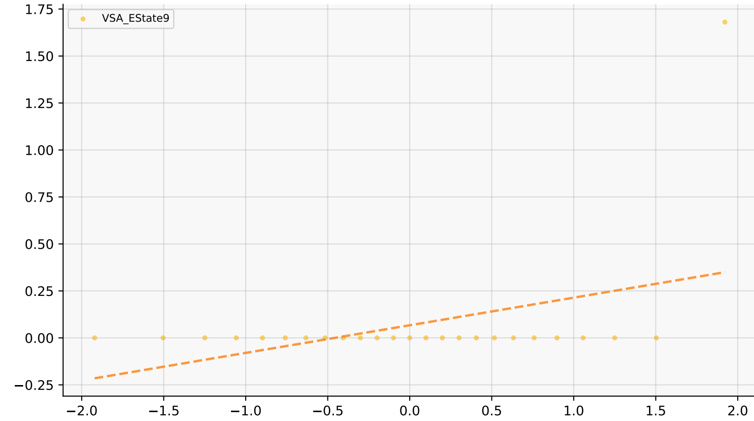
fr_methoxy
