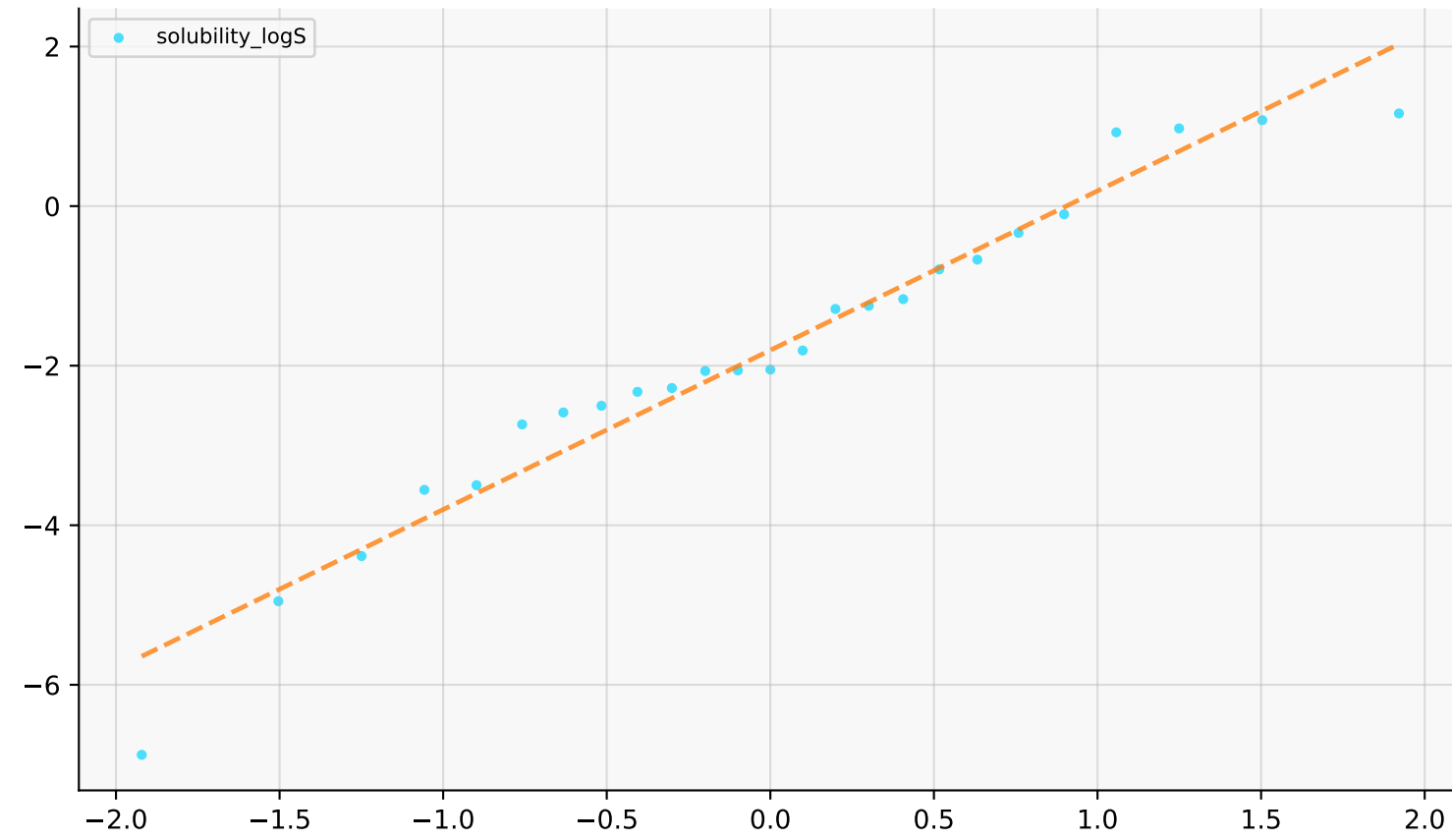
RDKitFP_1960
