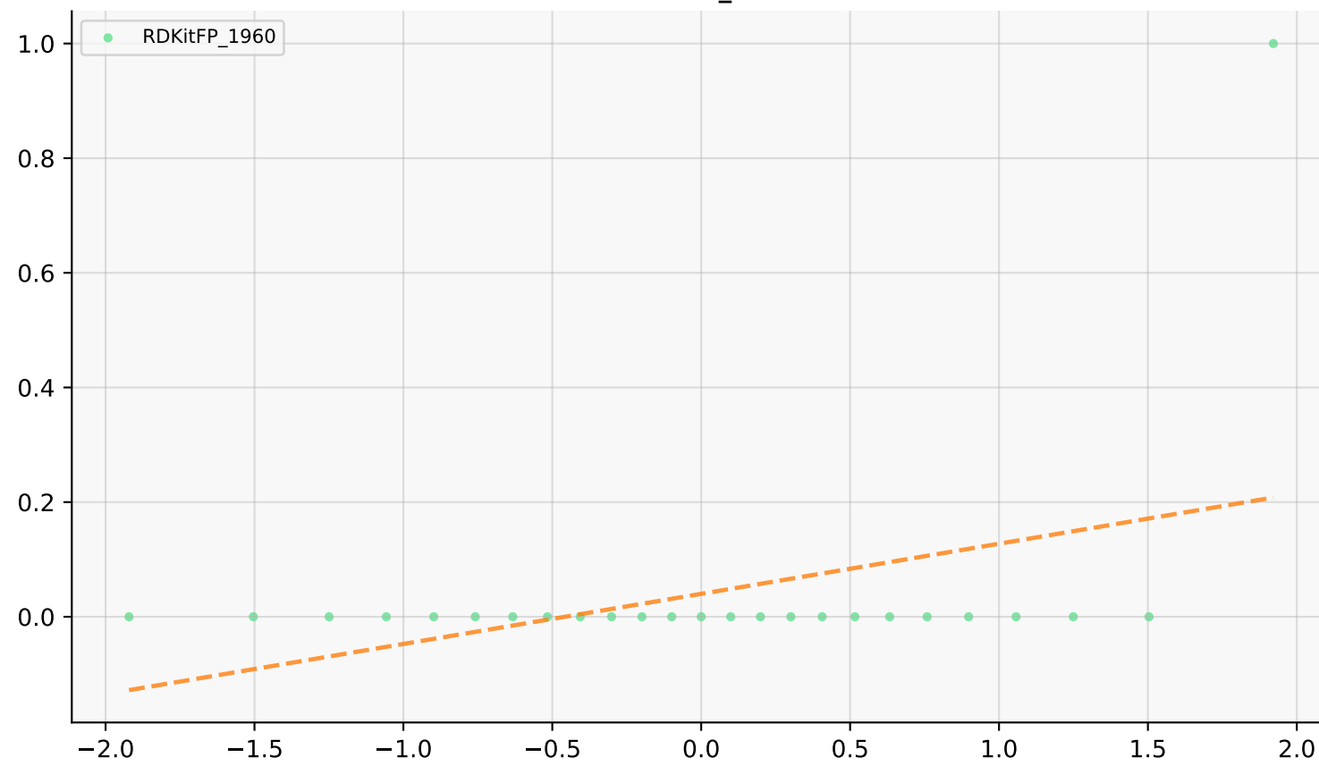
RDKitFP_1960
