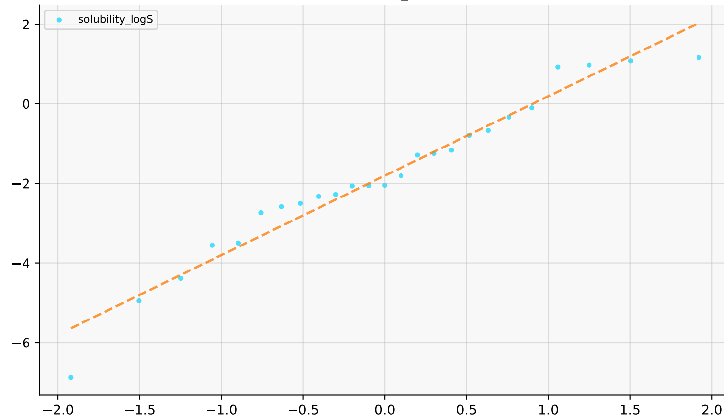
RDKitFP_1960
