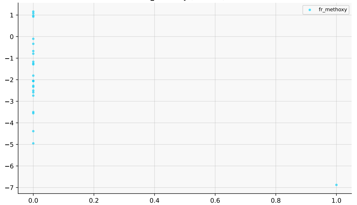
Morgan_r2_841 (r=-0.54)
