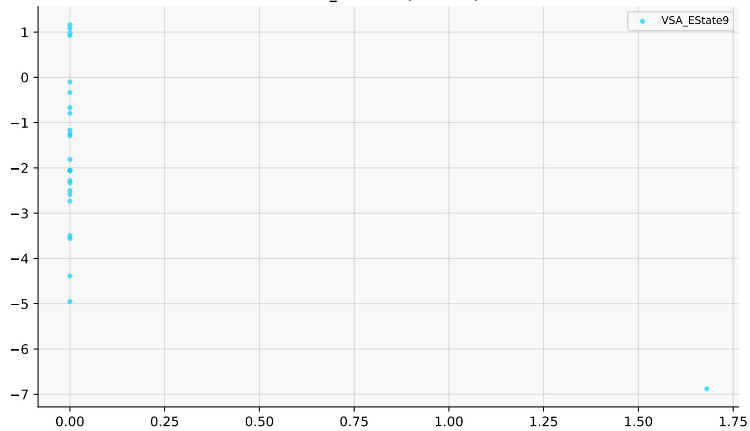
fr_methoxy (r=-0.54)
