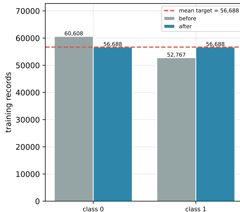
NSL-KDD (seed 42)
