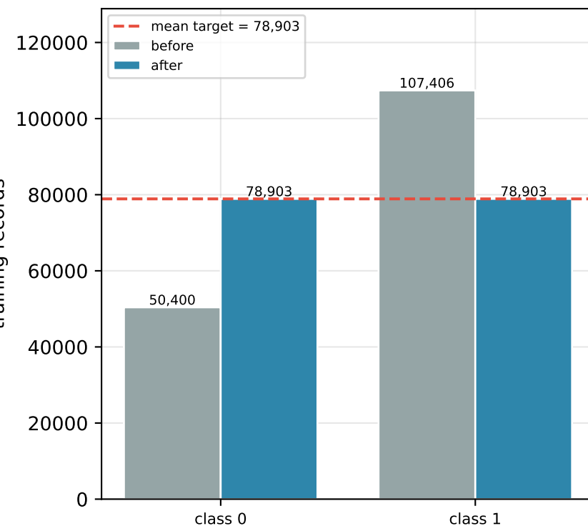
UNSW-NB15 (seed 42)
