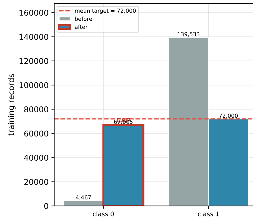
CIC-DDoS2019 (seed 42)
