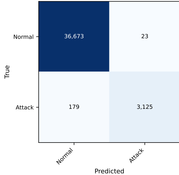
w/o Diffusion
