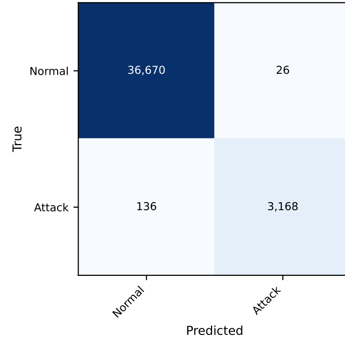
Baseline
