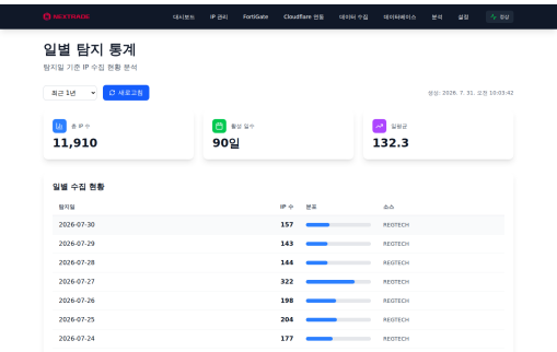
Figure 4: 분석
