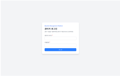
Figure 1: 로그인
