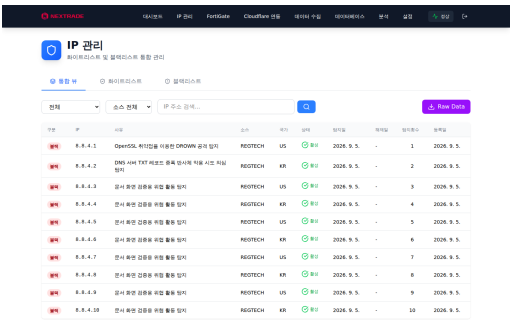
Figure 3: IP 관리
