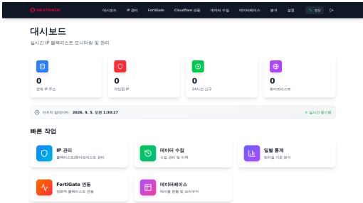
Figure 2: 대시보드
