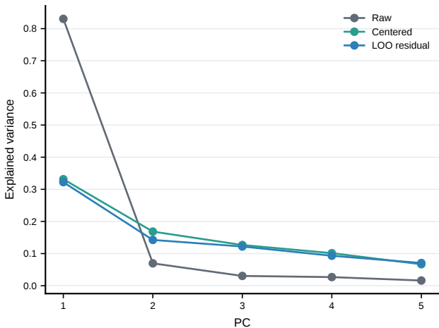
CGT axis PCA spectrum
