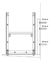
FIJACIÓN L EN FACHADA
