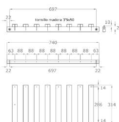
FIJACIÓN L EN FACHADA
