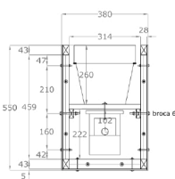
SECCION PANELES A-C
