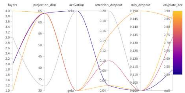
(a) Hiperparámetros de imagen contra precisión en validación
