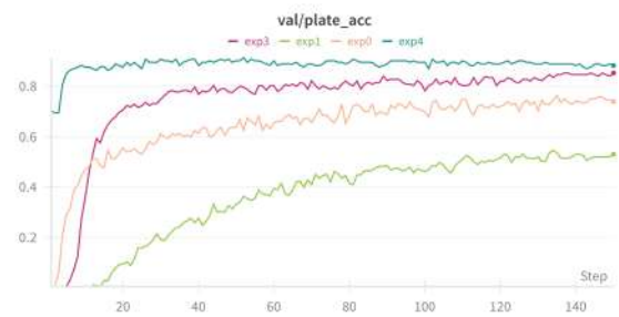
(d) Precisión durante validación
