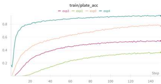
(c) Precisión durante el entrenamiento
