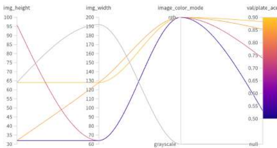
(a) Hiperparámetros de imagen contra precisión en validación
