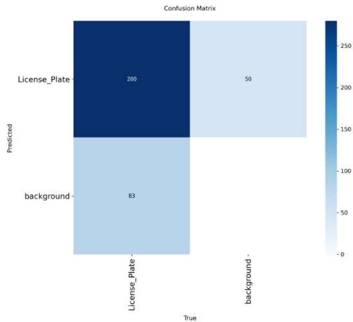
Figura 2: Desempeño del modelo original ante imágenes de varios países
