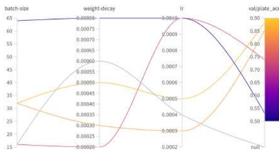
(c) Hiperparámetros del entrenamiento contra precisión en validación
