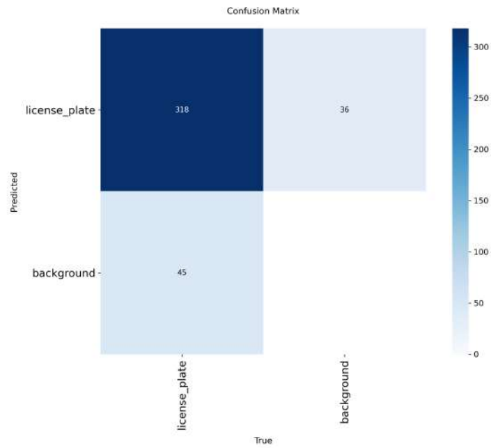
Figura 1: Desempeño del nuevo modelo ante imágenes de varios países
