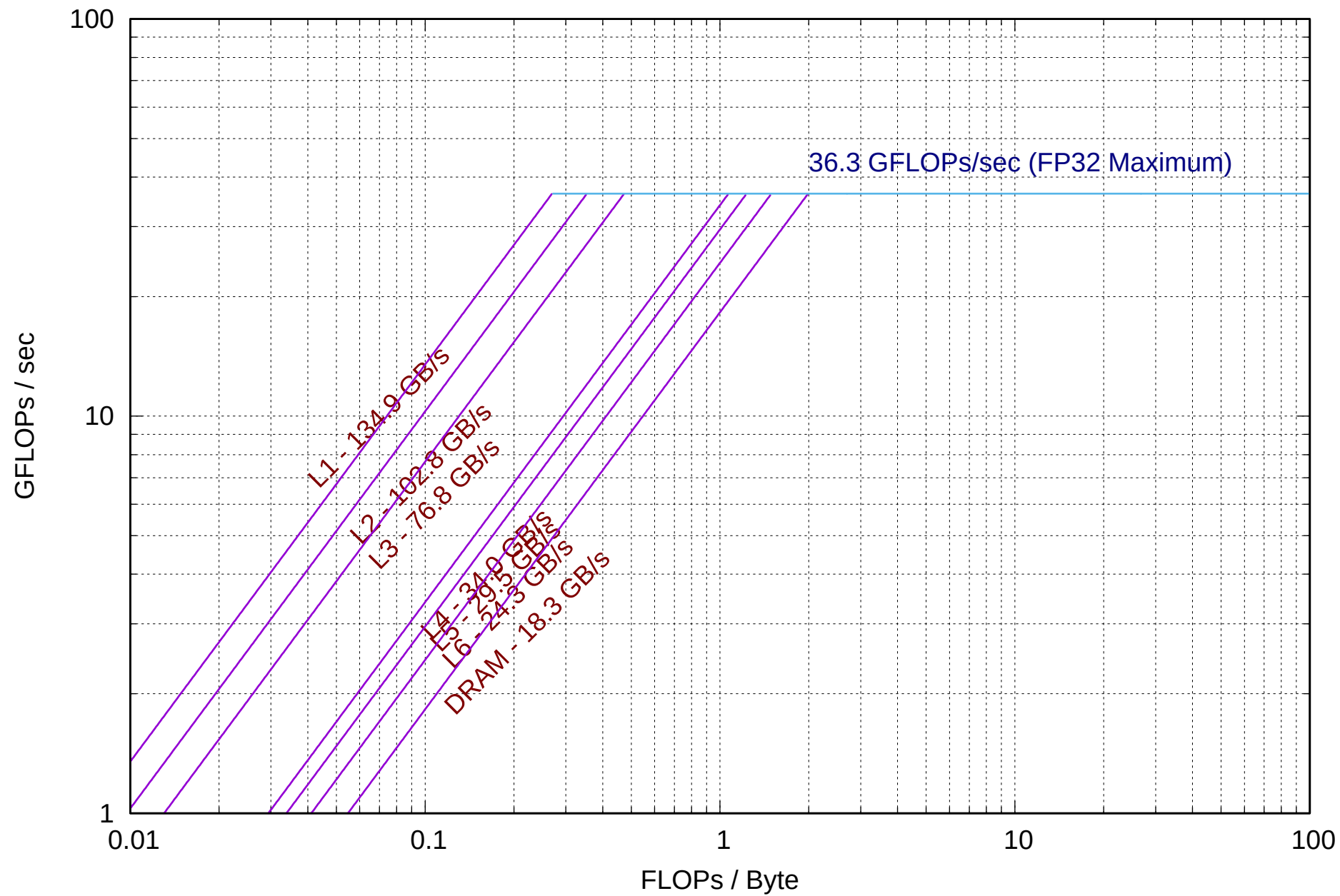
Empirical Roofline Graph (Resultados.desktop/Run.001)
