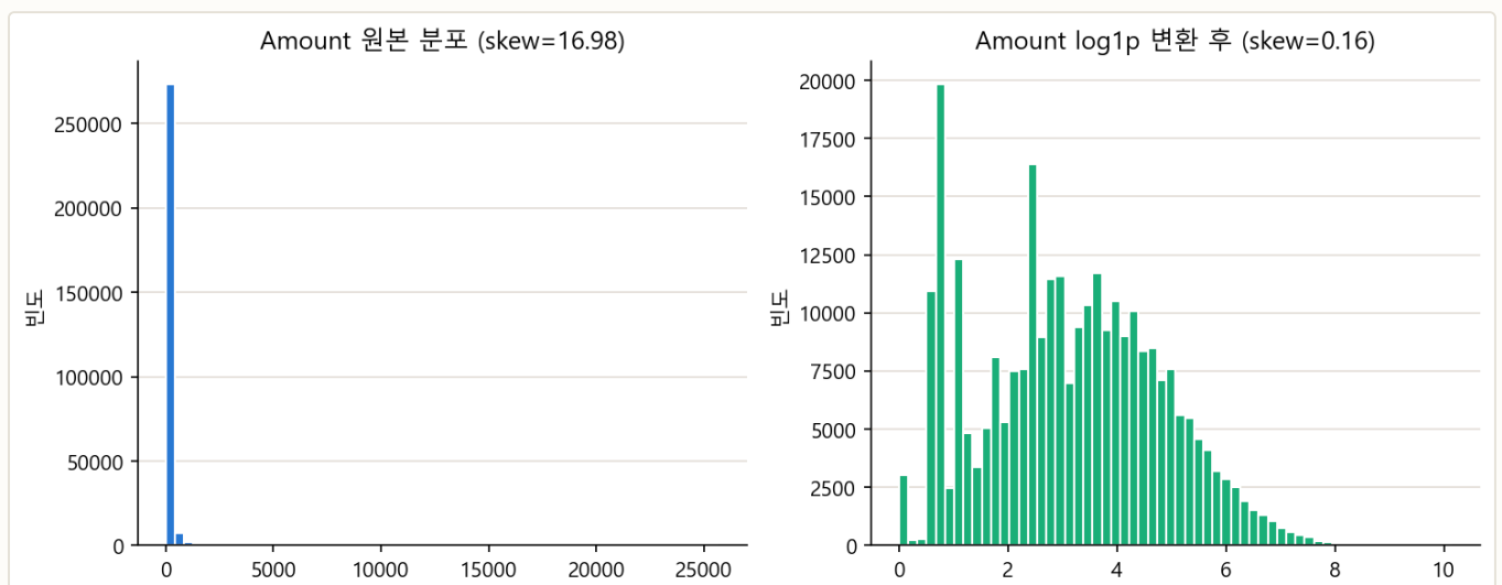
그림 3-2. Amount 원본(왜도 16.98) vs log1p 변환 후(왜도 0.16).
