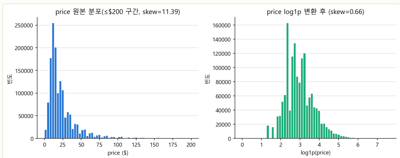
그림 5-1. price 원본 분포(≤$200 구간, 왜도 11.39) vs log1p 변환 후(왜도 0.66).
