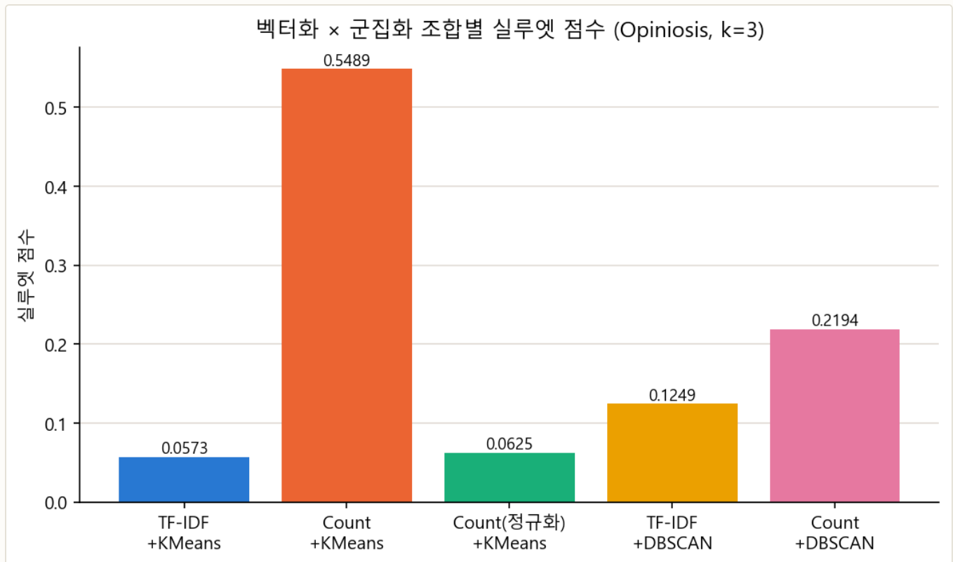
그림 4-1. 벡터화x군집화 조합별 실루엣 점수 비교(k=3).
