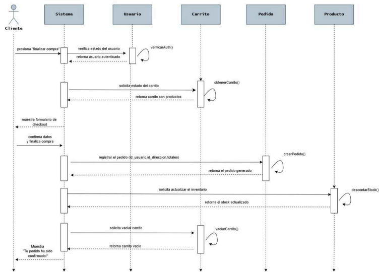
DIAGRAMA DE SECUENCIA Caso de uso: CONFIRMAR PEDIDO Actor: Cliente Caso: Normal - El cliente finaliza la compra con éxito.
