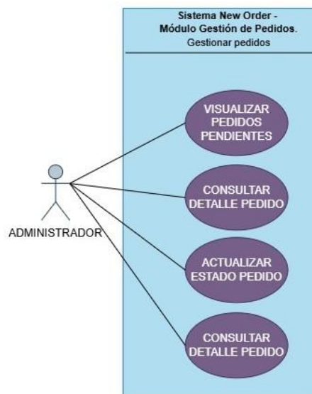
Figura 8: Diagrama de Casos de uso. Administrador-Gestionar pedidos
