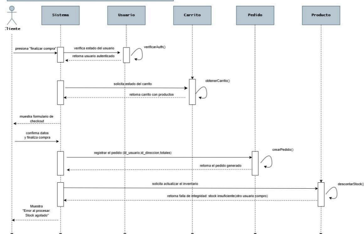
DIAGRAMA DE SECUENCIA Caso de uso: CONFIRMAR PEDIDO Actor: Cliente Caso: Alternativo 3 - Faltó de stock en la confirmación final. (qué pasa si otro usuario compra el último producto mientras vos estás en la pantalla de pago).
