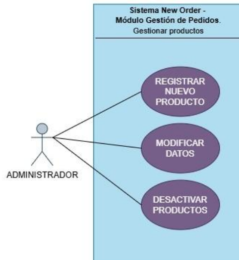
Figura 6 : Diagrama de Casos de uso. Administrador-Gestionar productos
