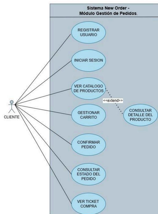
Figura 2: Diagrama de Casos de uso. Cliente
