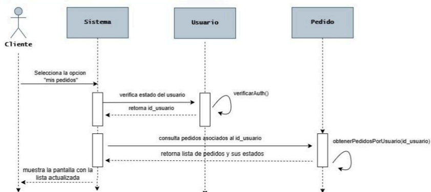
DIAGRAMA DE SECUENCIA Caso de uso: CONSULTAR ESTADO DEL PEDIDO Actor: Cliente Caso: Normal- Se encuentran pedidos asociados al id_usuario.
