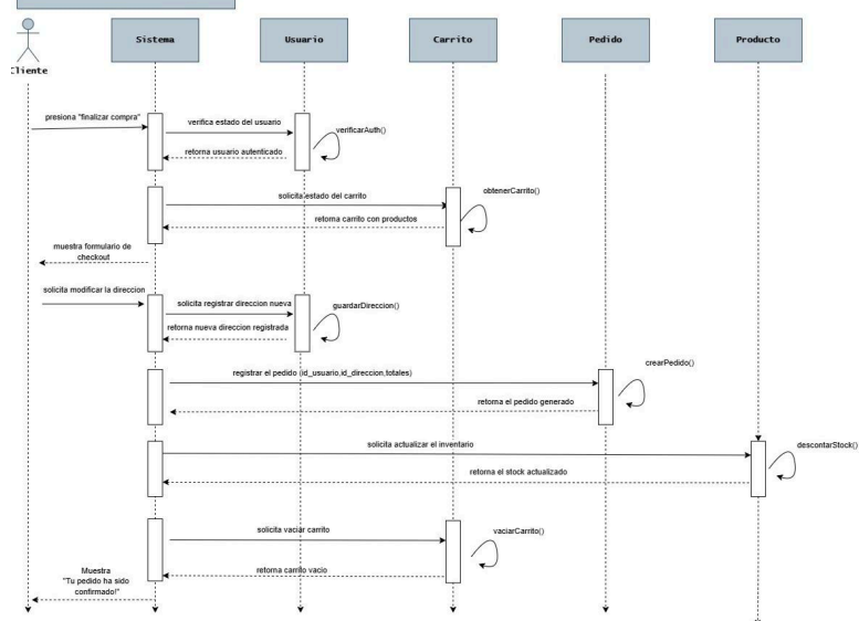
DIAGRAMA DE SECUENCIA Caso de uso: CONFIRMAR PEDIDO Actor: Cliente Caso: Alternativo 4 - Modificar direccion.
