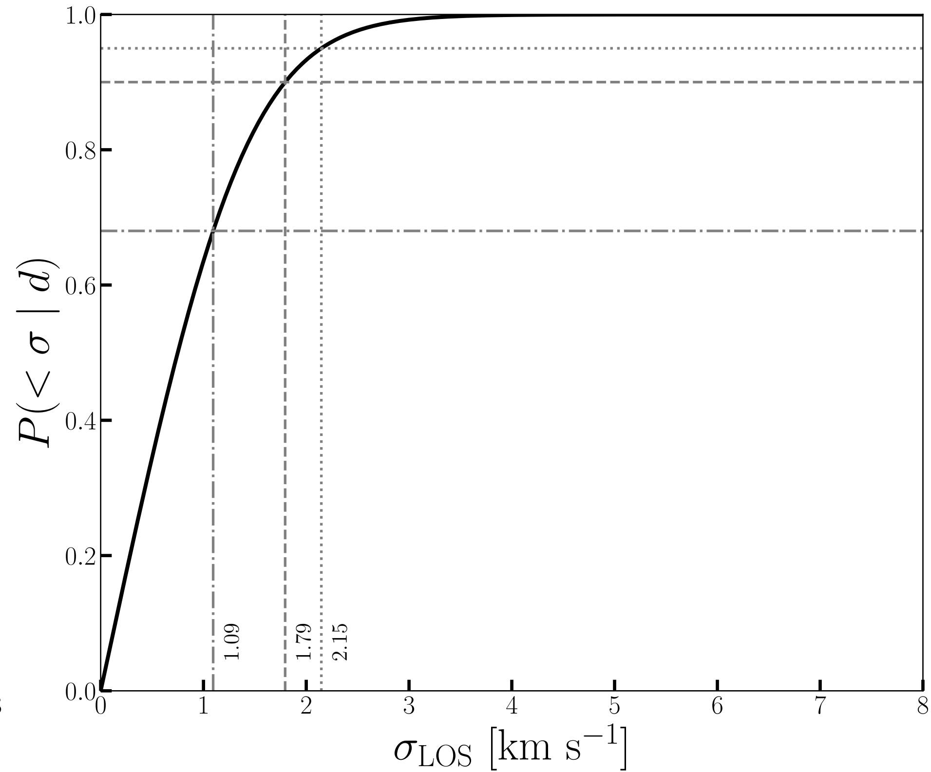
Segue2 (25 stars, LOS only) – velocity dispersion posterior
