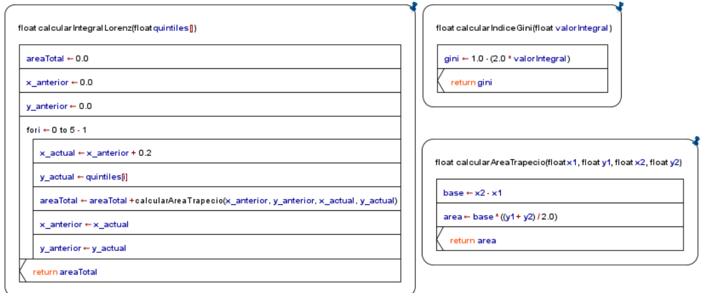
Figura 3. Diagramas Nassi-Schneidermann de los módulos matemáticos principales: calcularIntegralLorenz() , calcularIndiceGini() y calcularAreaTrapezio() .
