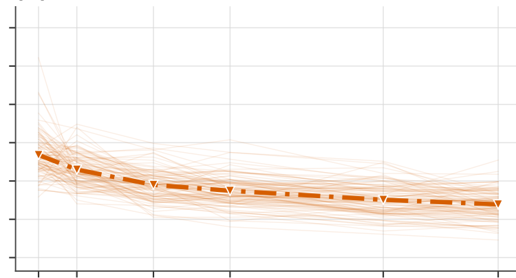
(D) AttnRelNet
