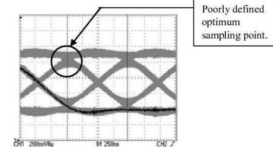
그림 12-4. 왜곡된 눈(eye) 다이어그램
