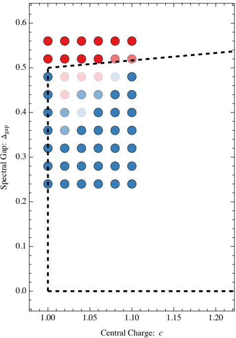
Integer Degeneracy, \Delta_{\max}=3
