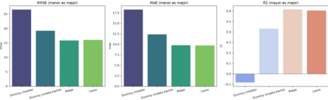
Comparativa de modelos baseline
