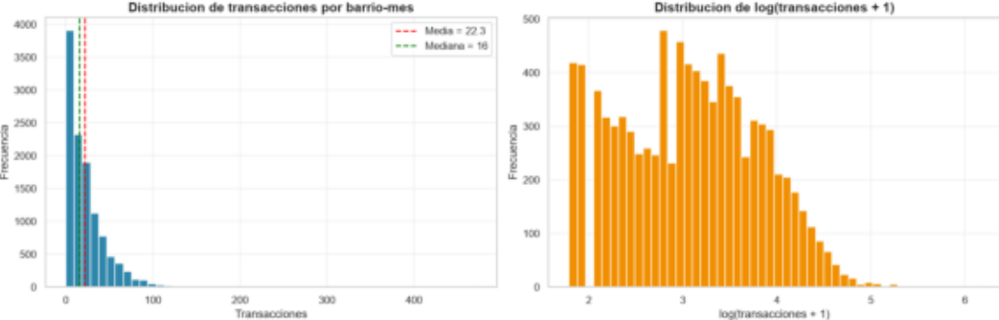
Distribución del target (skewness = 2,76)
