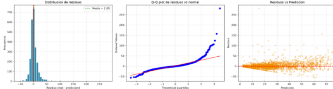
Análisis de residuos del modelo
