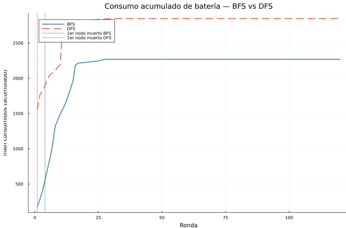
Figura 16: Consumo acumulado total BFS vs DFS
