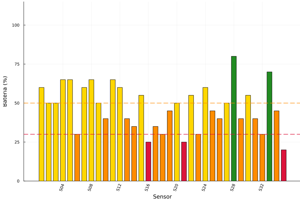
Figura 8: Estado de batería todos los sensores
