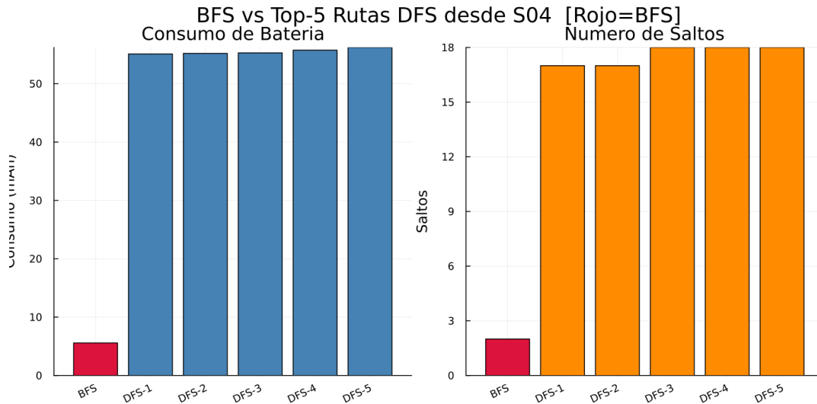
Figura 7: Comparación BFS vs top-5 rutas DFS
