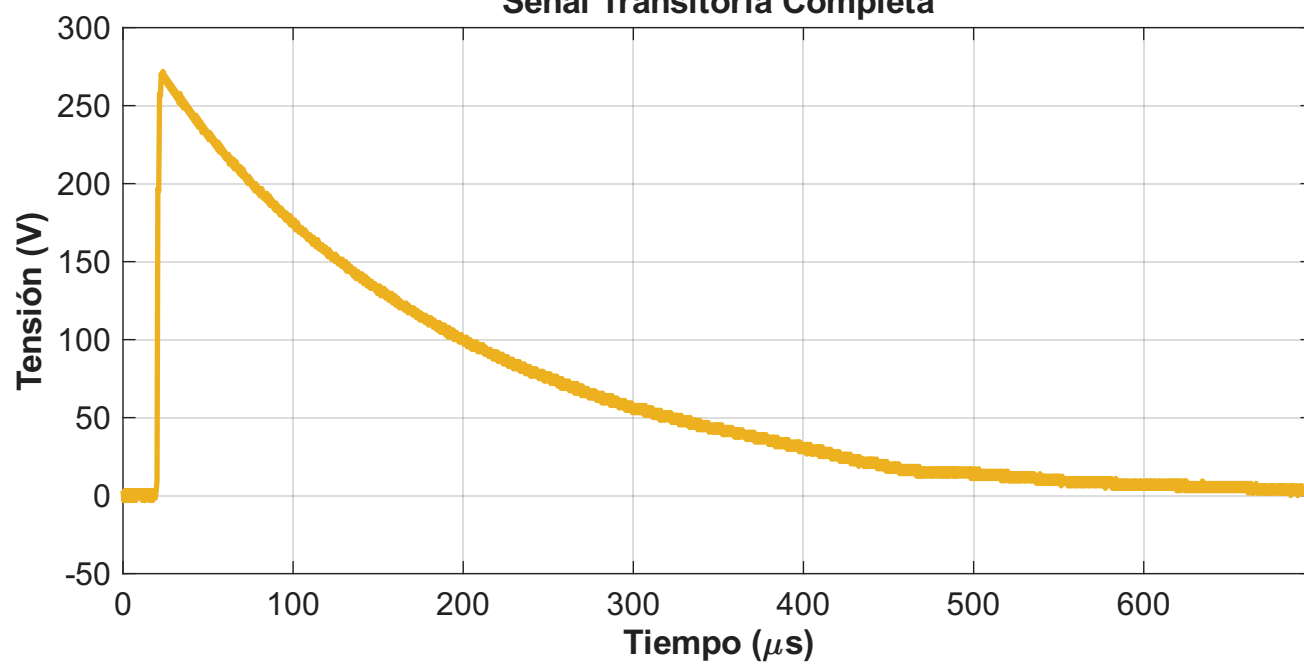
Señal Transitoria Completa
