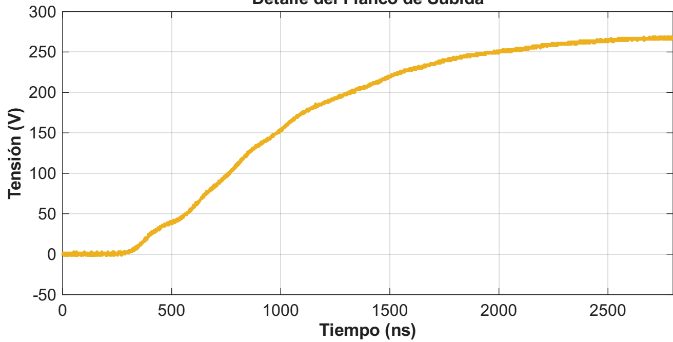
Detalle del Flanco de Subida
