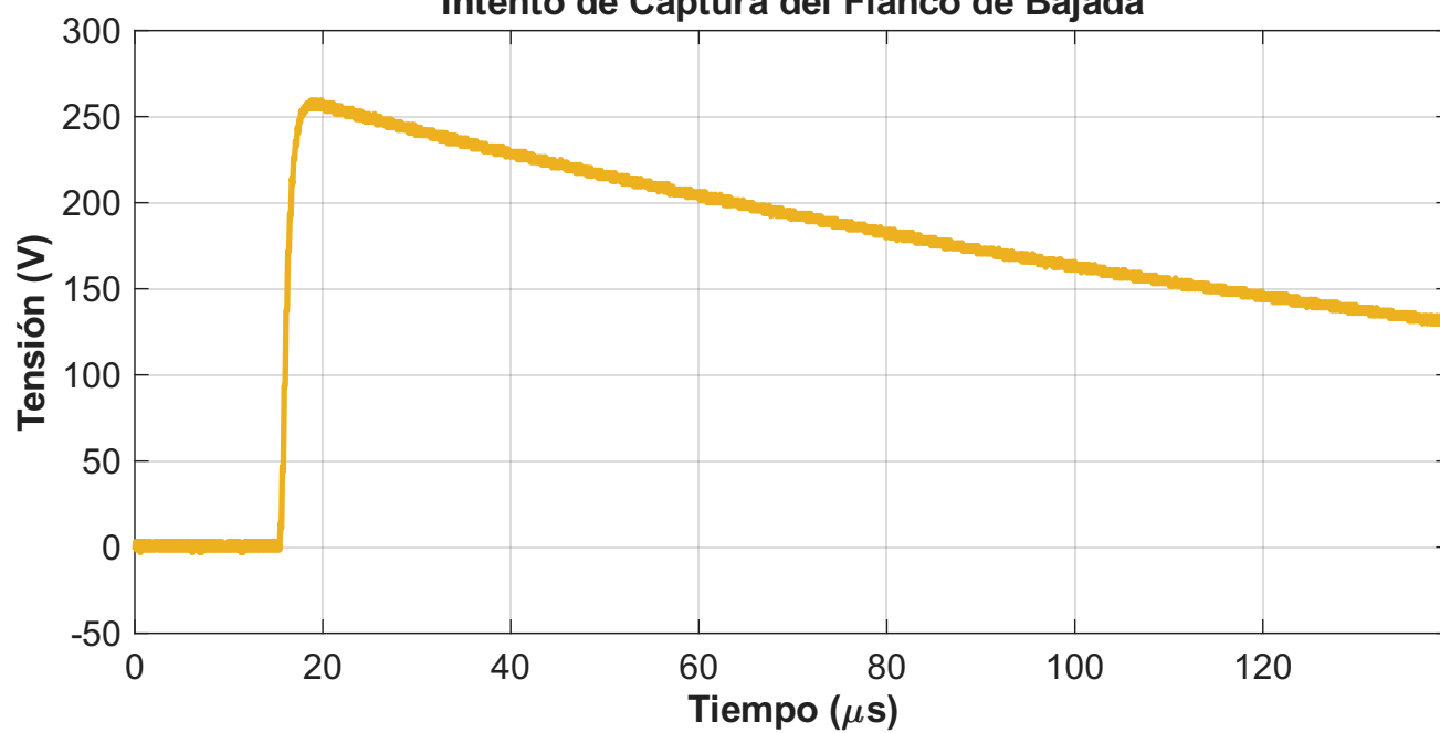
Intento de Captura del Flanco de Bajada
