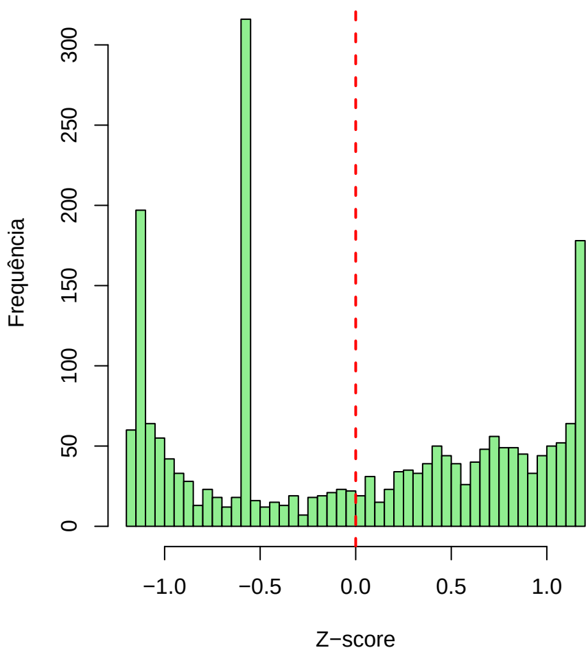
Distribuição dos Z-scores
