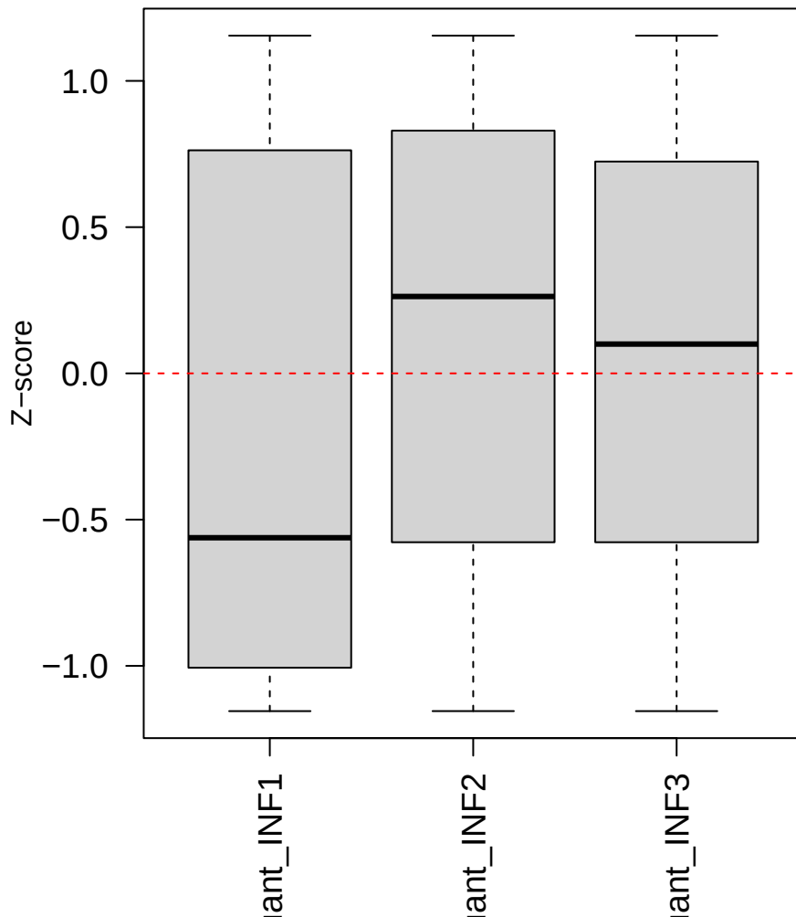
Z-scores por Amostra
